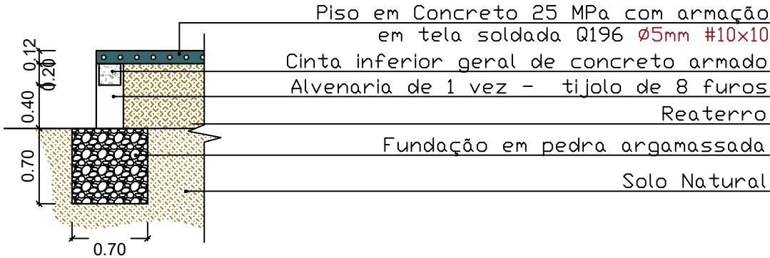
Detalhe – Corte escala 1/50
