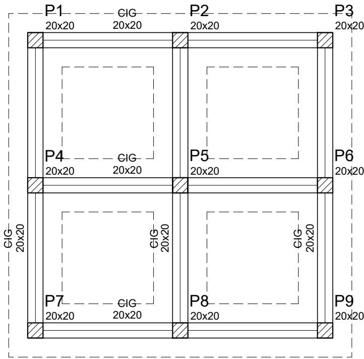
Forma Base de Reservatório Inferior escala 1/50
